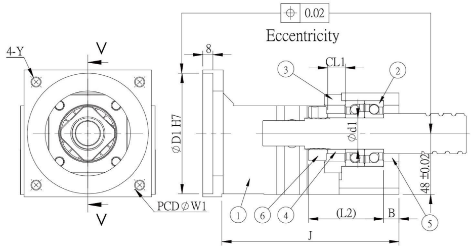
Section V-V
